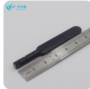
YW-698/2700-5D-160mm
