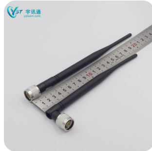
YW-800/2100-5D-Nmale
