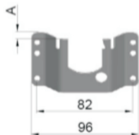
Support a legno per 405.712... Aufschraublager für 405.712... Bearing Bracket for 405.712... 405.712...系列配套支架
