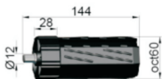
Calotta oct60 con perno \varnothing 12 Kapsel oct60 mit stift \varnothing 12 Plastic cap oct60 with pivot \varnothing 12 塑料尾插, oct60, 配 \varnothing 12 的销子
