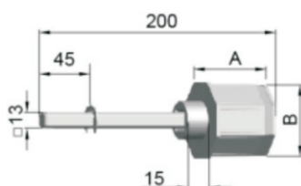
Calotta registrabile in alluminio(reg.max=90mm) Verstellbare kapsel aus aluminium(verst.max=90mm) Adjustable Aluminum Idler(max.adj=90mm) 可调式铝合金尾插 (最大调节长度=90mm)
