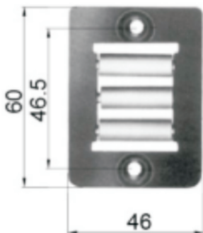
Guidacinghia tre rulli per Omega Gurfführung mit drei Rollen FÜR OMEGA Strap guide with three rollers for Omega OMEGA 用导轮
