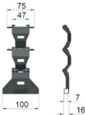
Superblock per Stecca "Maxi" Superblock für stäbe: "Maxi" Superblock for slat: "Maxi" 通用型大帘片防上推
