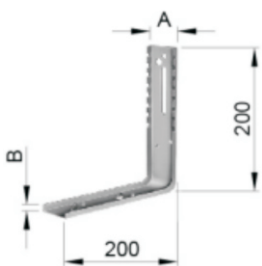
Parte verticale per support"TORINO"90° Vertical Arm for Torino Supports,90° bended直角端端支架
