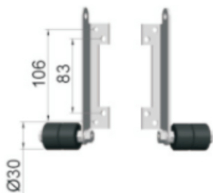
Rullino d'invito Dx e SIN, Per Fianchi 250,300 Paar Einlaufrollen, für Groß e blendkappen 250,300 Entry Guide Roller, for End Cap 250,300,large leg 引导轮, 配套250, 300的大尺寸腿端盖使用
