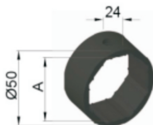
Rullo In Ferro E Accessori Achtkantwellen Und ZubehÖre Octagonal Tube 八角管
