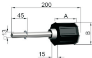
Calotta registrabile zincata(reg.max=90mm) Verstellbare stahlkapsel(verst.max=90mm) Adjustable steel cap(max.adj=90mm) 可调式铁尾插 (最大调节长度=90mm)
