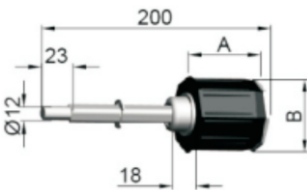
Calotta registrabile zincata(reg.max=90mm) Verstellbare stahlkapsel(verst.max=90mm) Adjustable steel cap(max.adj=90mm) 可调式铁尾插 (最大调节长度=90mm)
