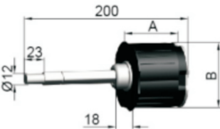
Calotta registrabile zincata(reg.max=90mm) Verstellbare stahlkapsel(verst.max=90mm) Adjustable steel cap(max.adj=90mm) 可调式铁尾插 (最大调节长度=90mm)
