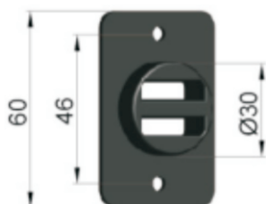
Guidacinghia vert.in pladtica per Omega Senkrechte Gurtführung aus Kunststoff FÜR OMEGA Vertical plastic strap guide for Omega OMEGA 用双扁导口 (立式)
