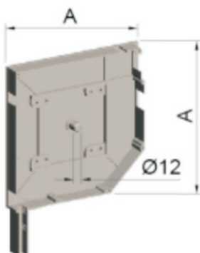
Paia di fianchi(DX e SN)45° Per motore, con pemo Ø12 Paar blendkappen(rechts und links)45° für der motor,mit stiff Ø12 Pair of End Cap 45° for fubular motor,with pivot Ø12 45° 管状电机用铝端盖,带Ø12的柱子
