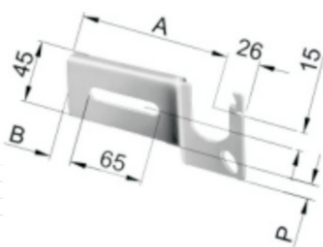
Mensole per supporti TORINO DESTRA Bracket for Torino supports right 冲压轴承支架, 右
