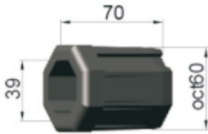
Adattatore oct40/oct60 Aufsteckringe oct40/oct60 Plastic Adapter, oct40/oct60 塑料转换适配件, oct40/oct60
