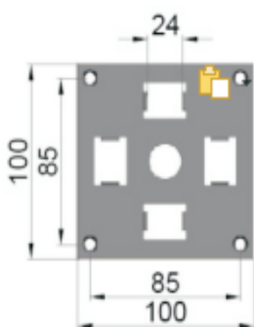
Piastra per fianchi Lagerplatte für Gro ß e blendkappen Support plate for king size end caps 管状电机安装座
