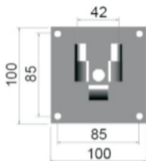
Piastra per fianchi Lagerplatte für Gro ß e blendkappen Bracket for bearing OD42 for king size end caps 外径42轴承支架
