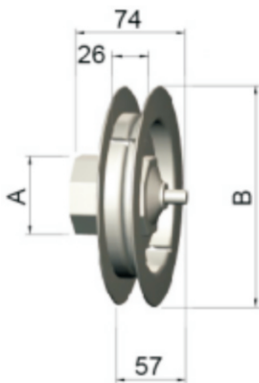
Puleggia in ferro con perno Ø12 Stahlgurtscheibe mit sfiiff Ø12 Steel pulley with pivot Ø12 铁轮盘, 带Ø12的销子
