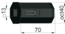
Calotta in plastica oct40 con foro 13 Kunststoff Walzenkapsel oct40 mit loch 13 Plastic cap oct40 with Hole 13 塑料尾插, 40八角管用,带13*13mm方孔
