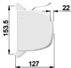
Avvolgitore a bandiera con/per cintino Mini-Gurtwickler Mit/fÜR Gurt Strap Coiler 带式收绕盒
