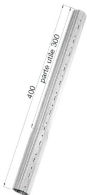
Prolunga(corsa 250mm)zincata Teleskopwelle(lauf 250mm) Tube Extension(stroke 250mm) 异形八角管 (可调节行程 250mm)
