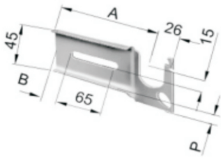
Mensole Rovesciate per supporti TORINO DESTRA Bracket for Torino supports right(reverse) 冲压轴承支架，右
