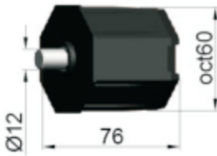
Calotta oct40 con perno Ø12 Kapsel oct40 mit stift Ø12 Plastic cap oct40 with with pivot Ø12 塑料尾插, oct460,配Ø12的销子
