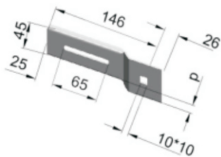
Mensola per supporti NAPOLI con foro ■ 10 Bracket for NAPOLI supports with hole ■ 10 NAPOLI 10mm单方孔支架
