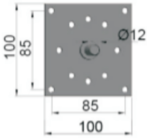
Piastra per fianchi Lagerplatte für Gro ß e blendkappen Support plate for king size end caps 支撑板
