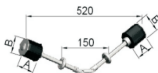
Caloffa doppia registrabile con snodo cardanico Verstellbare doppelkapsel mit Kardangelenk Double-Adjustable Plastic Idler,with cardan joint 双头45°可调式塑料过渡尾插
