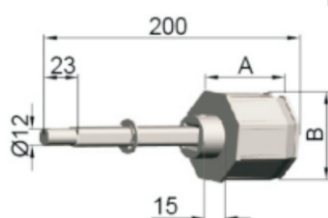
Calotta registrabile in alluminio(reg.max=90mm) Verstellbare kapsel aus aluminium(verst.max=90mm) Adjustable Aluminum Idler(max.adj=90mm) 可调式铝合金尾插 (最大调节长度=90mm)
