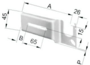
Mensole Rovesciate per supporti TORINO SINISTRE Bracket for Torino supports left 冲压轴承支架（反向），左
