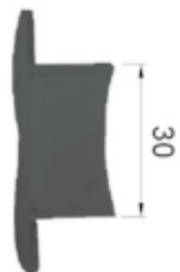
Calotta per stecca 37mm Kapsel für stäbe 37mm End cap for slat 37mm 37mm帘片用侧扣
