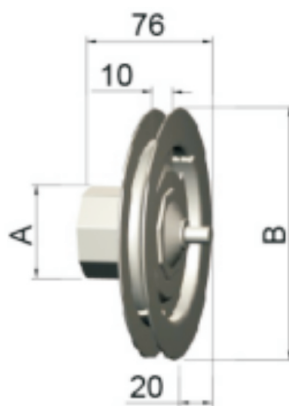
Puleggia in ferro con perno Ø28, per fune Stahlgurtscheibe mit sfiiff Ø28, für drahtseil Steel pulley with pivot Ø28, for steel wire 铁轮盘, 带Ø28的销子, 与钢丝绳配用
