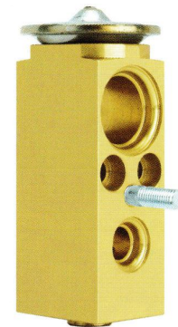
适用车型: 别克/福特 OE#:B-9117610 YX62309
