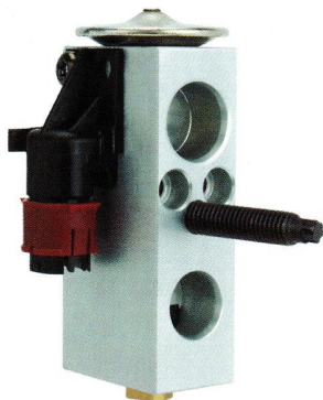
适用车型: 克莱斯勒 OE#:C-5019218AE YX62313
