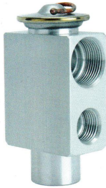
适用车型: 大众3000 参考号:E-321 501 YX62137
