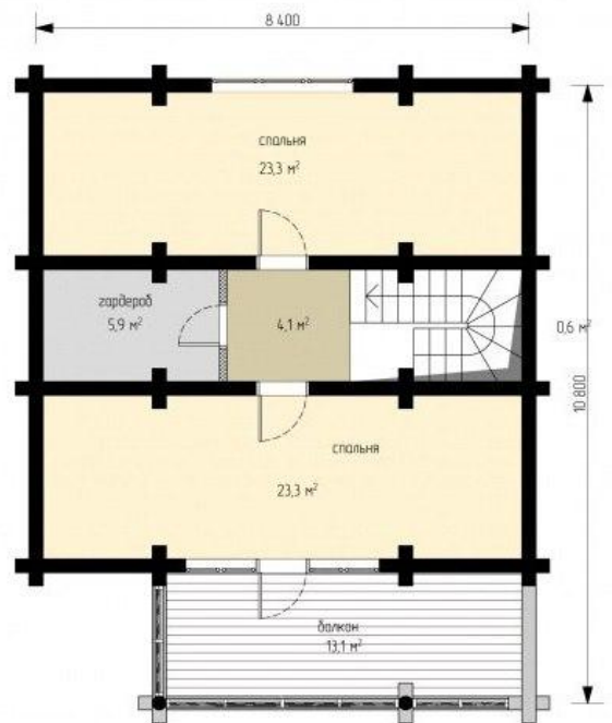
План 2 этажа
