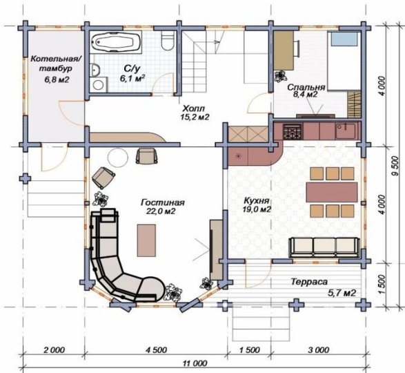
План 1 этажа
