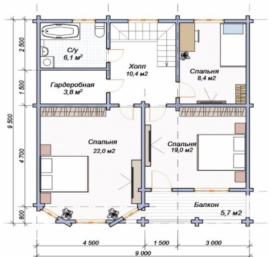
План 2 этажа
