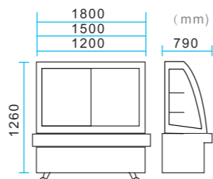
◀ XL-1200A1 / XL-1500A1 / XL-1800A1
