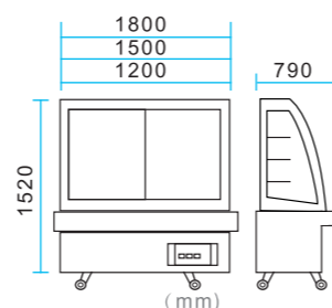
◀ XL-1200C / XL-1500C / XL-1800C
