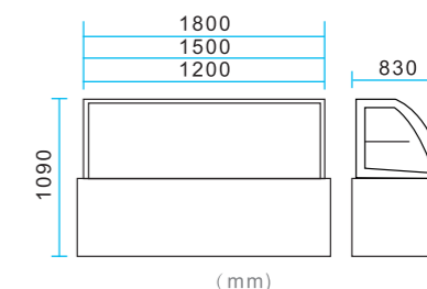
◀ XL-1200A2 / XL-1500A2 / XL-1800A2
